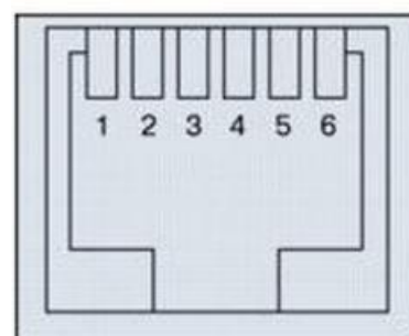
RS232Інтерфейс зв'язку
