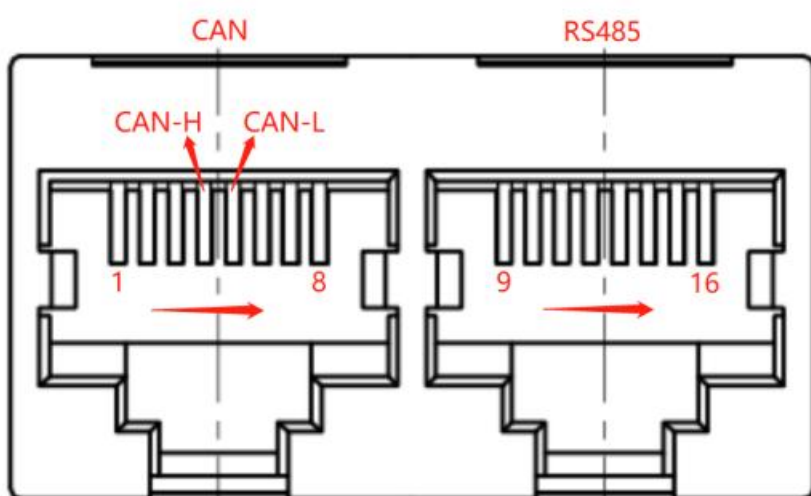
МОЖЕІRS485інтерфейс
